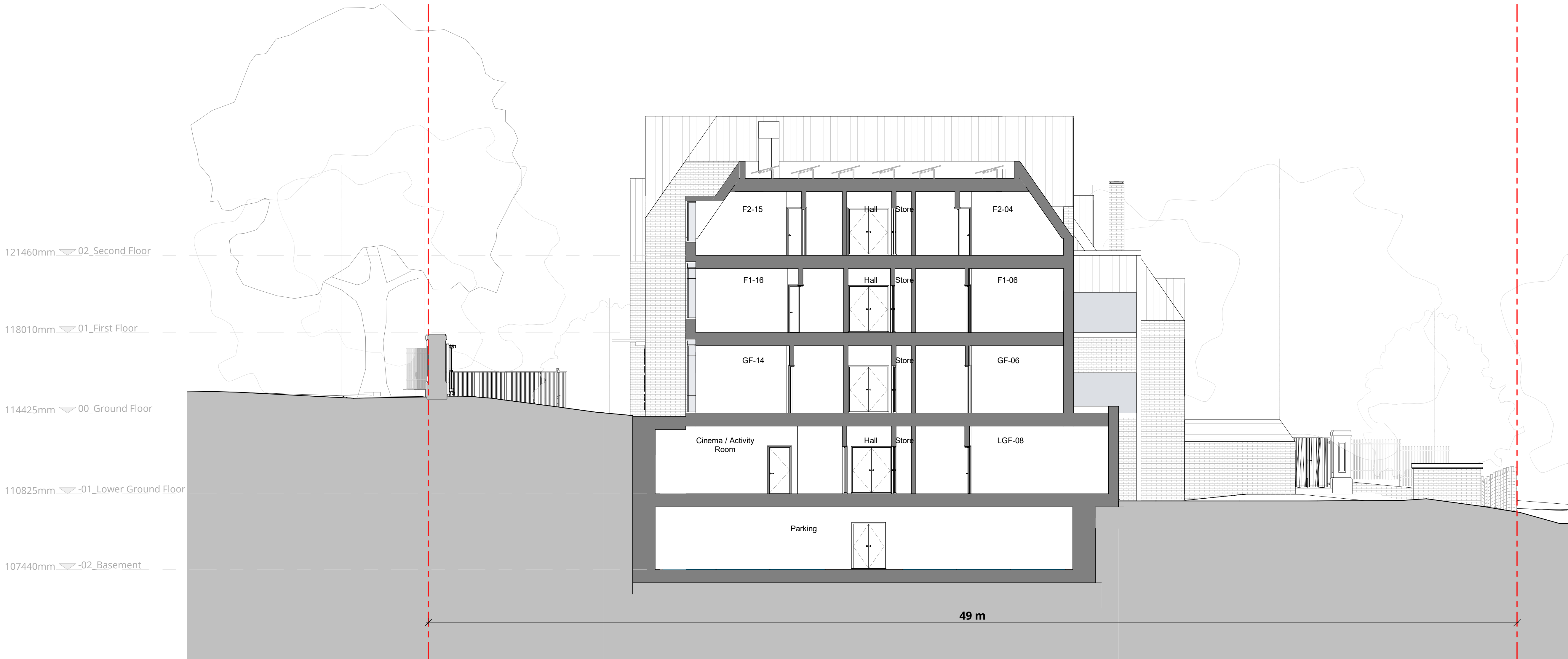
Section A-A 1:100
