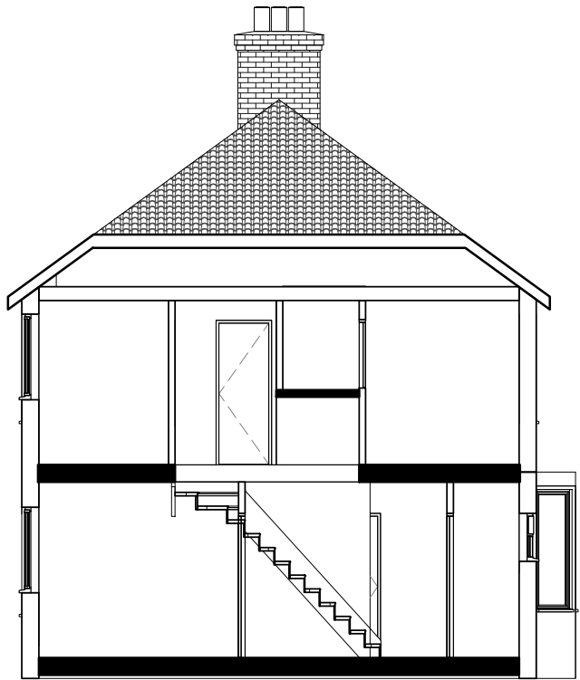
Section Existing 1 : 100
