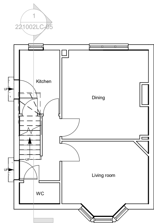
01. GF Existing 1 : 100
