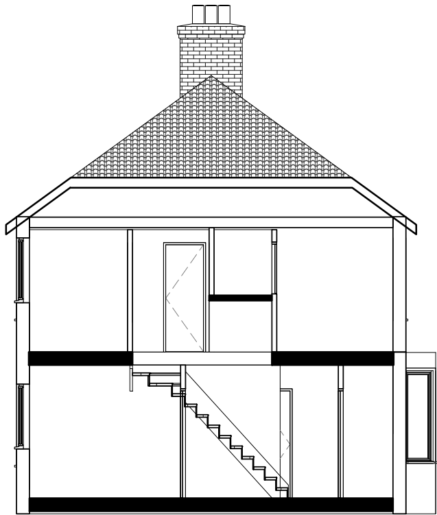
Section Existing 1 : 100
