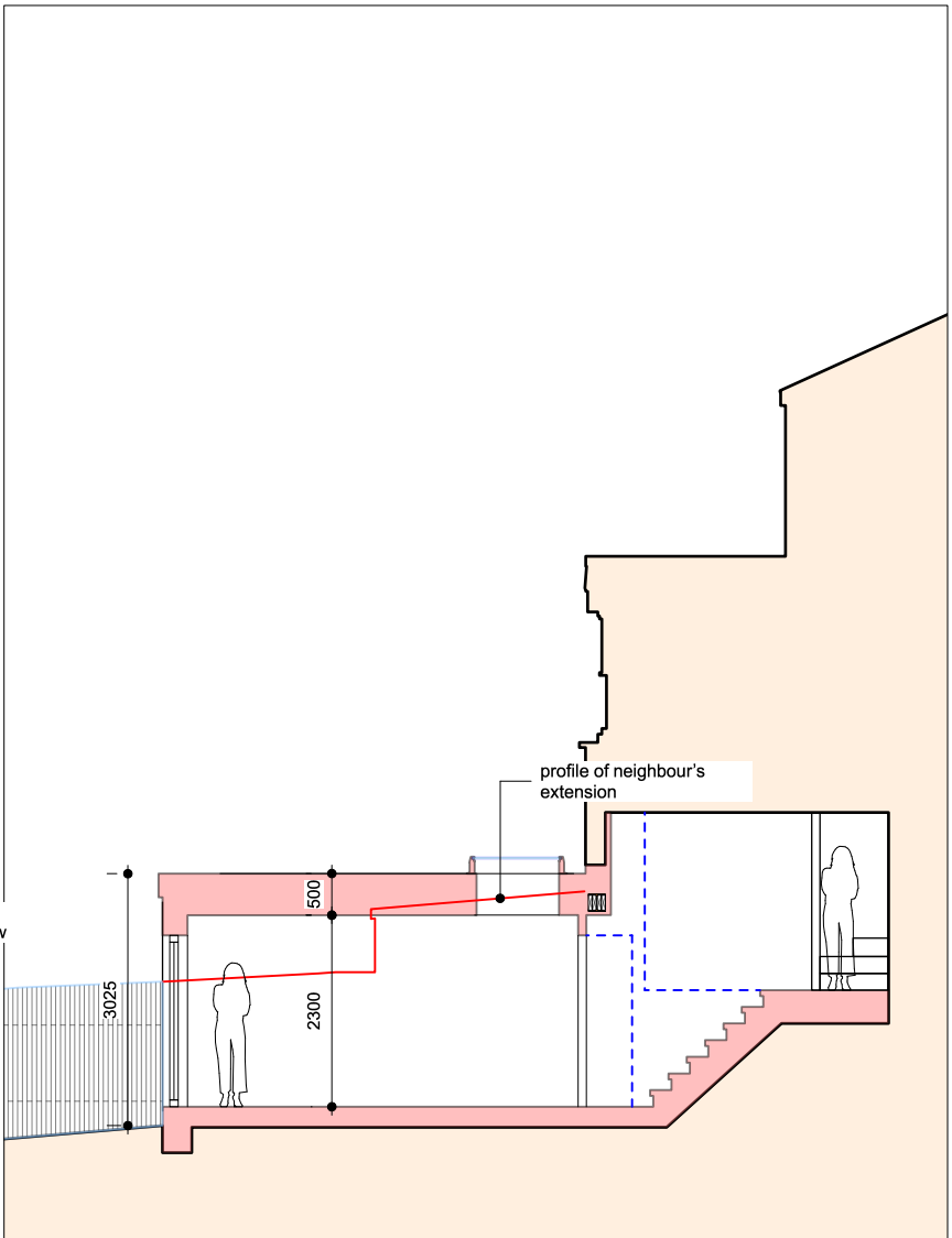
03 section a-a 1:100
