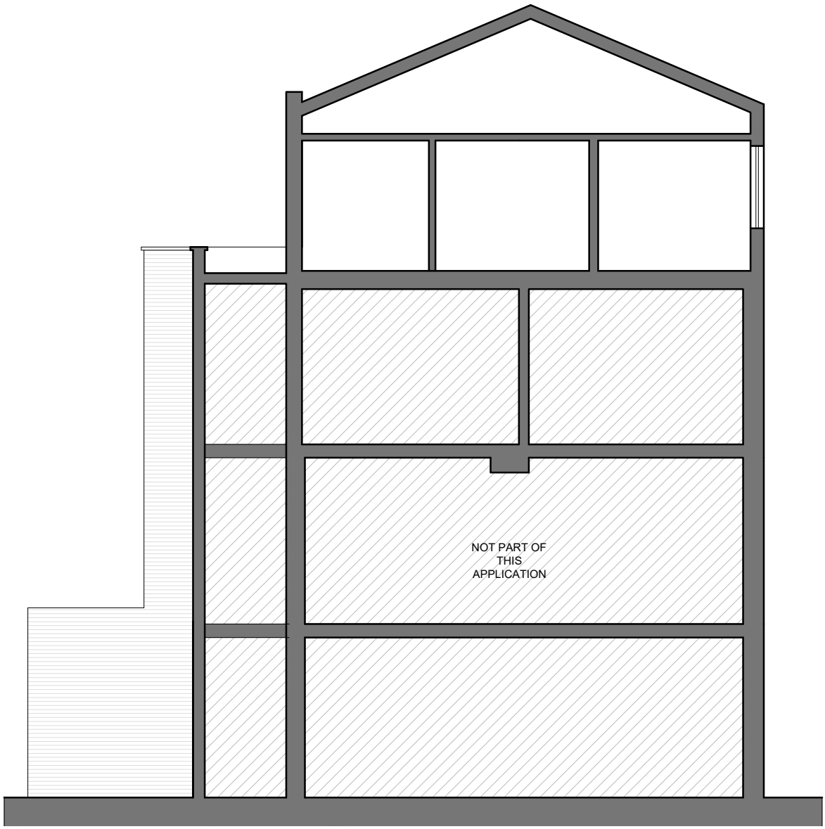
Existing Section BB 1:100 @ A3
