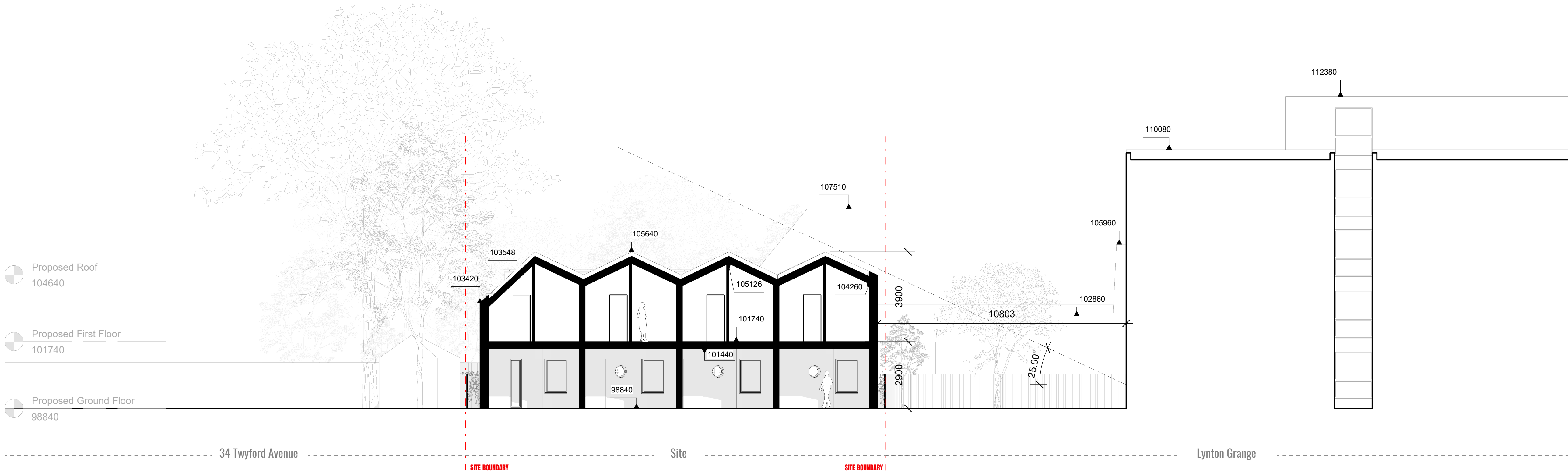
1 Section A-A 1:100
