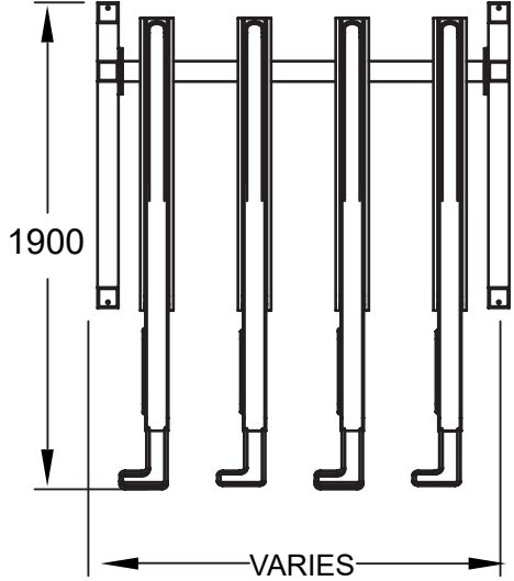
TOP
