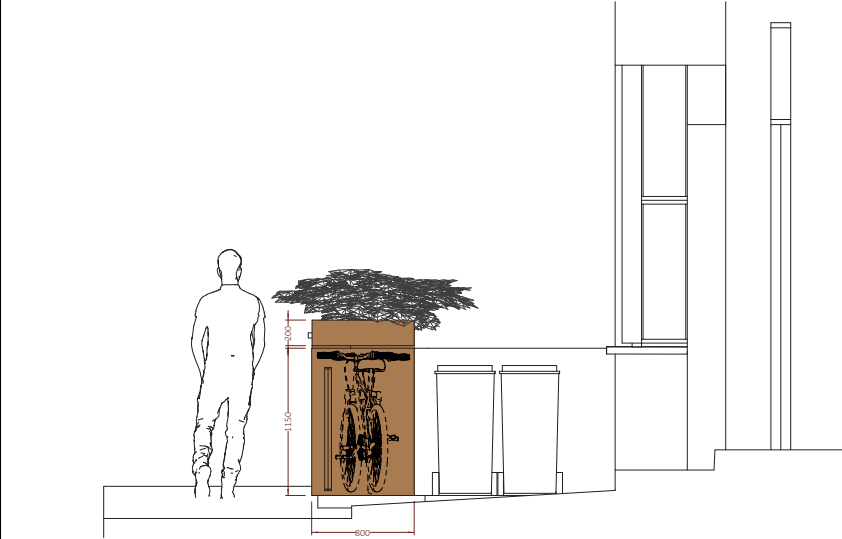
02 Elevation
