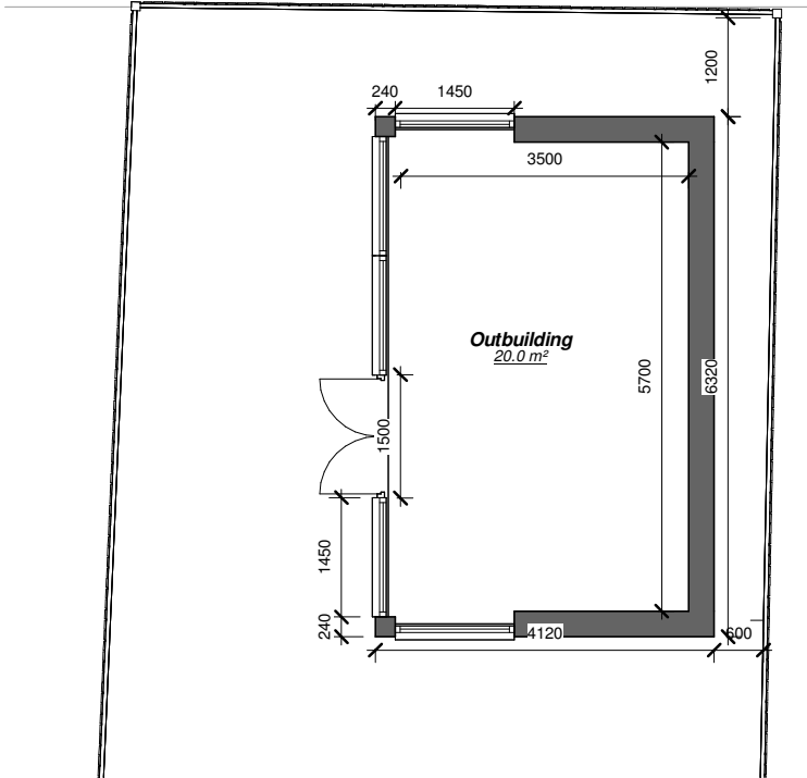
GF Lvl (O) 1 : 100
