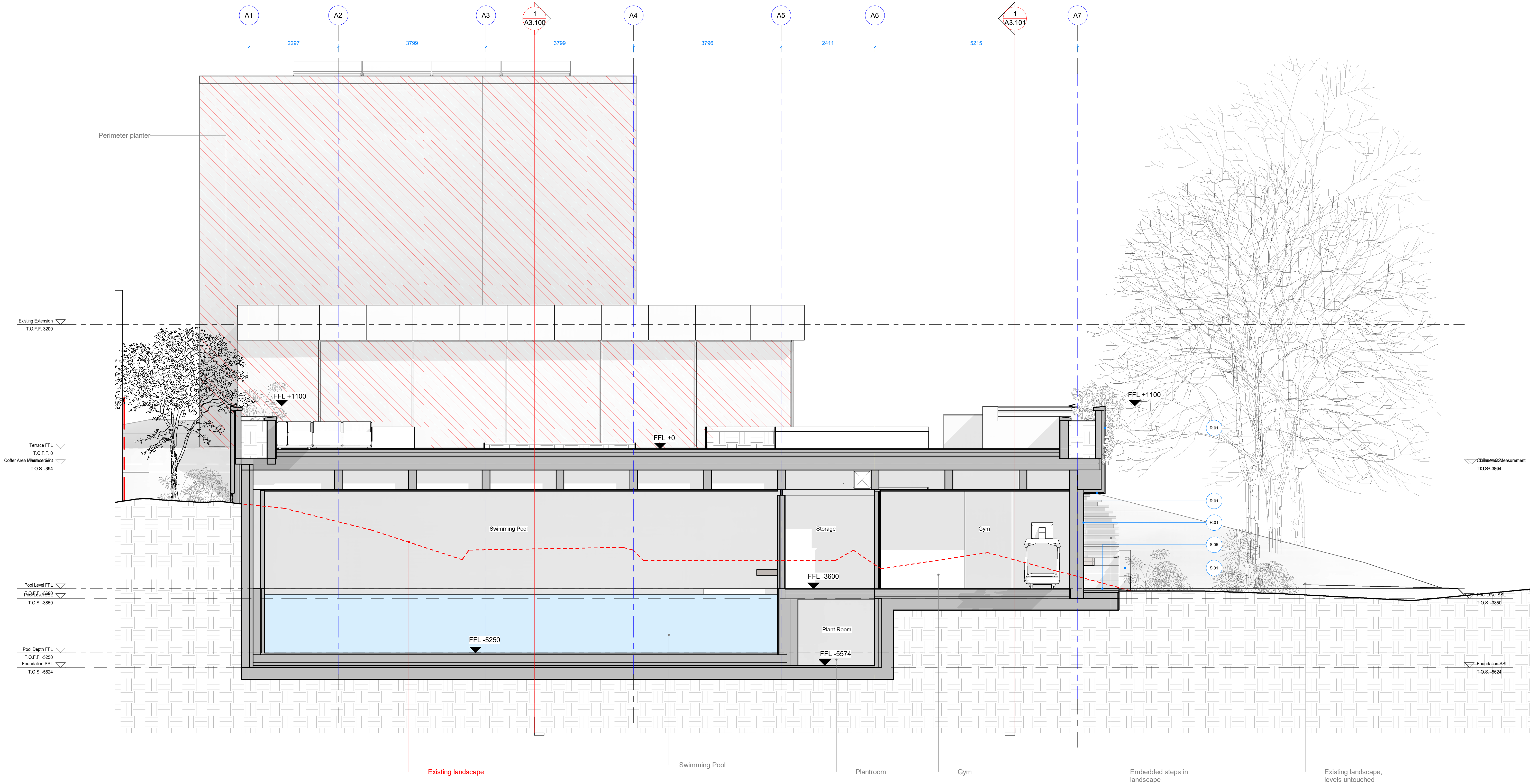
1 Section CC SCALE 1 : 50
