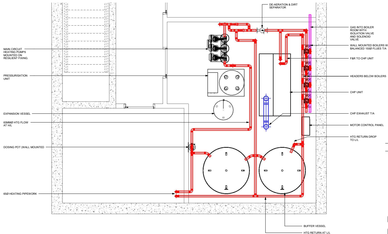
1 Basement Plan 1 : 25
