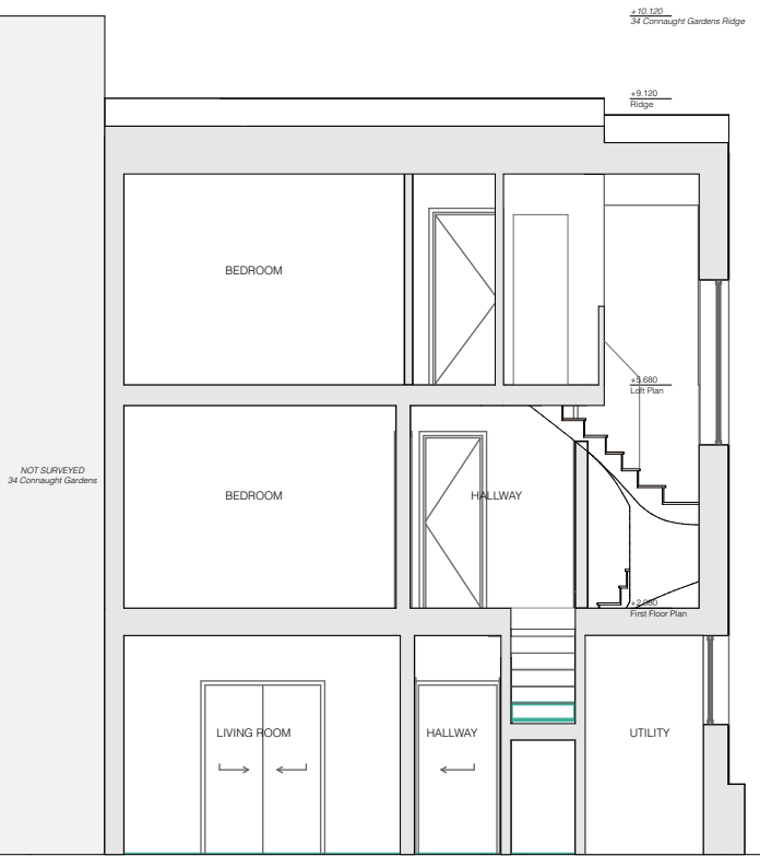
Section BB 1:100
