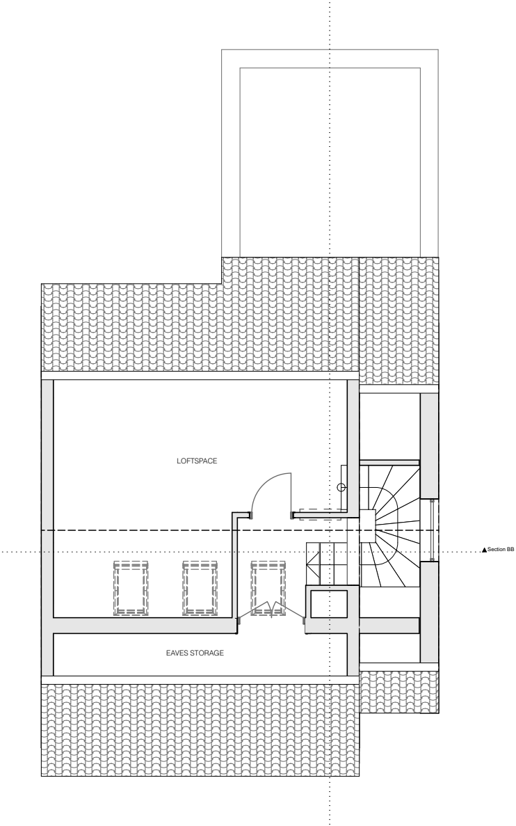
Roof / Loft 1:100
