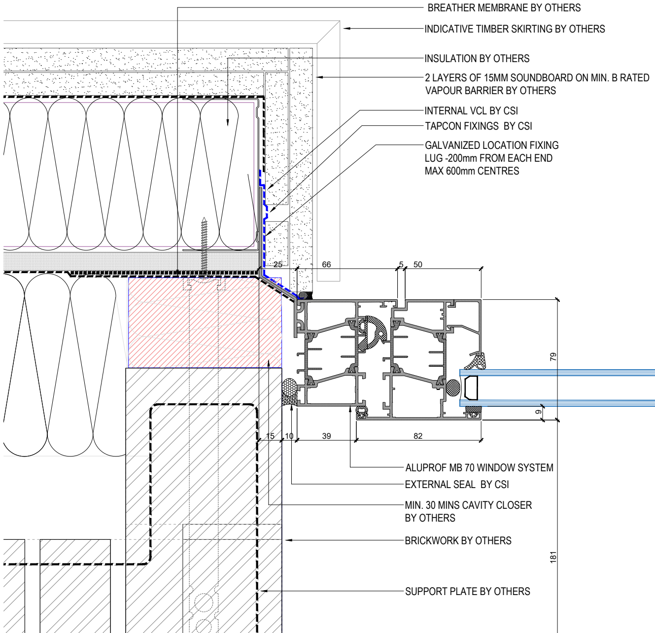
43 SECTION SCALE: 1:2.5
