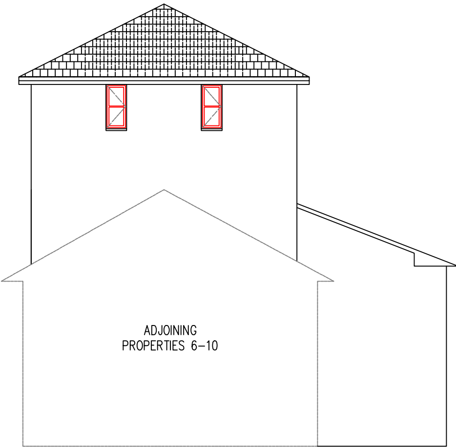
FLANK ELEVATION 1
