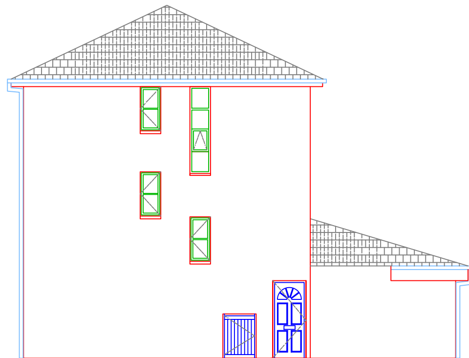
FLANK ELEVATION 1
