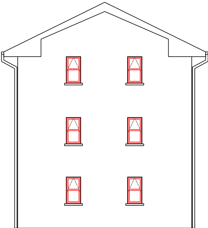
FLANK ELEVATION 2
