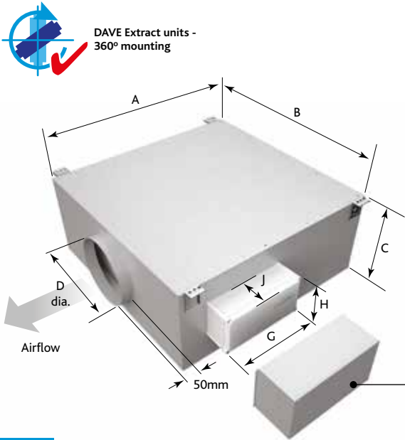
EXTRACT FAN SIZE DE3 - DIMENSIONS (mm)
