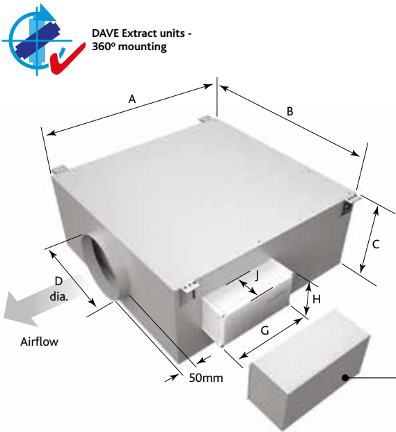
EXTRACT FAN SIZE DE7 - DIMENSIONS (mm)
