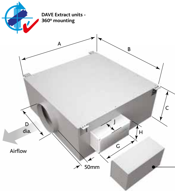
EXTRACT FAN SIZE DE2H - DIMENSIONS (mm)
