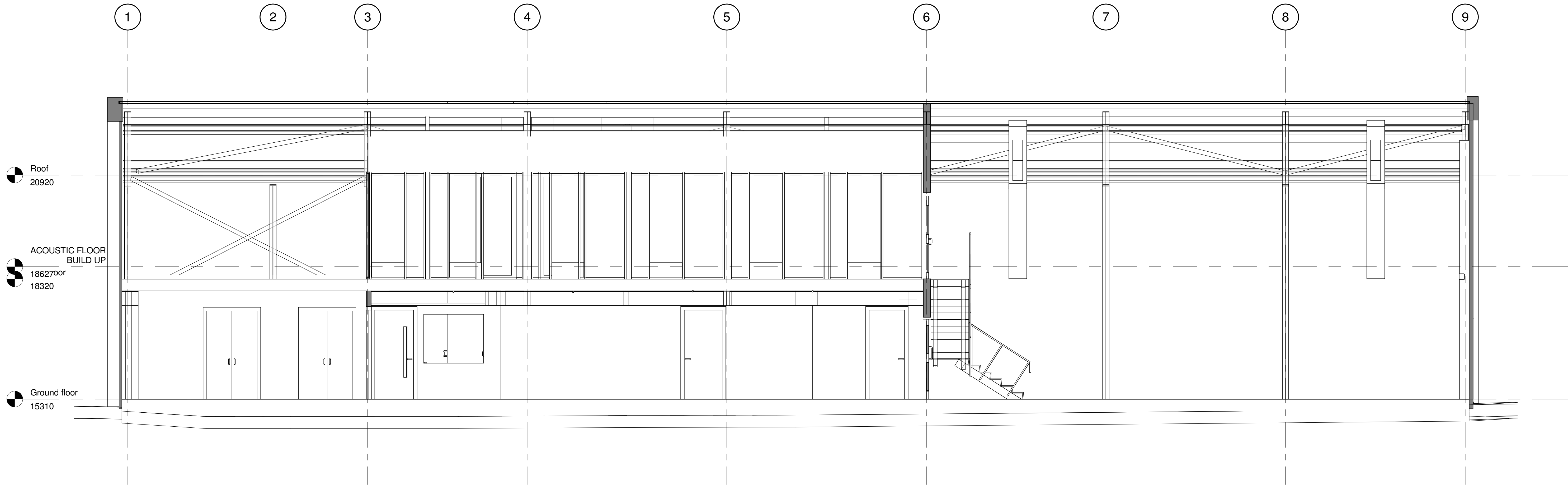
1 EXISTING LONG SECTION DD 1 : 50
