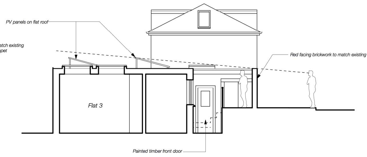
Section DD
