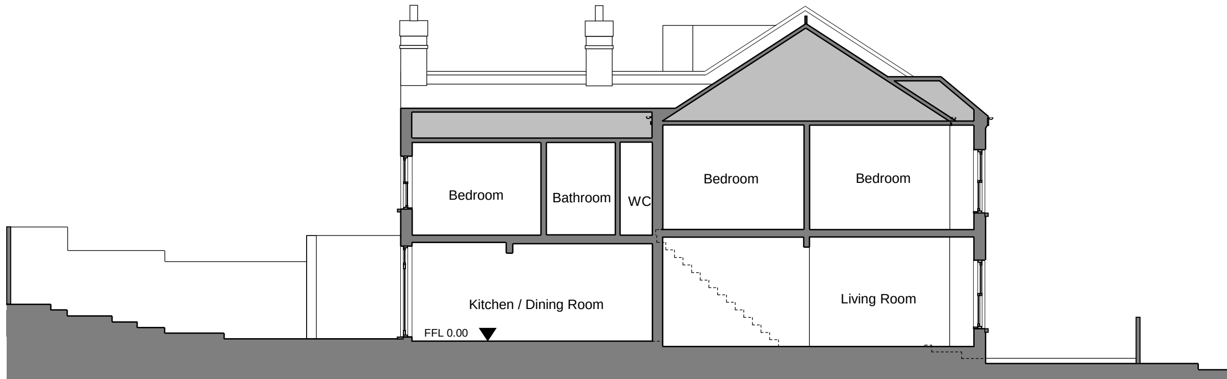
Section A-A
