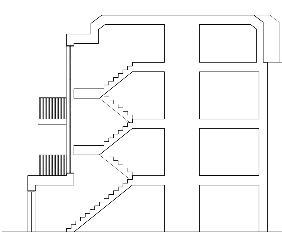
Section A-A
