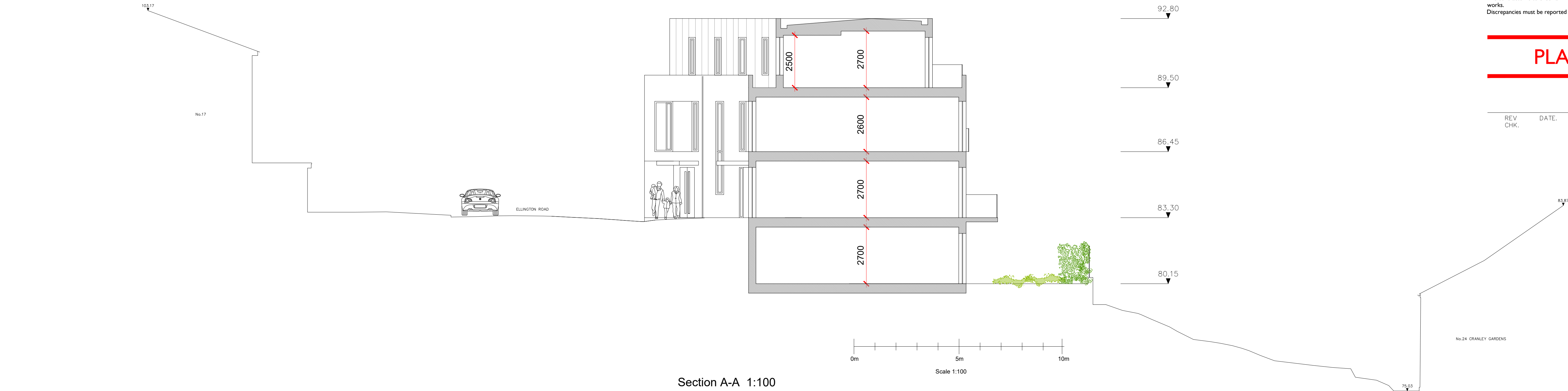
Section A-A 1:100
