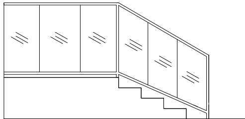
5 Stairs detail Scale: 1:50
