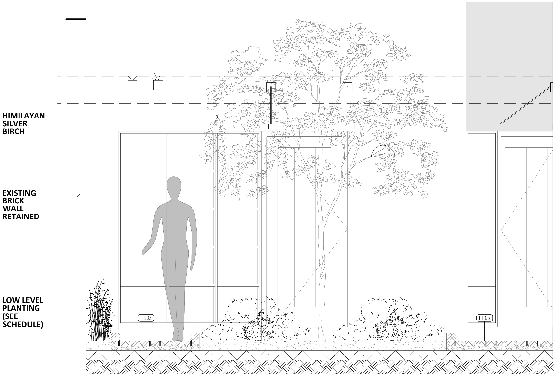
SECTION A-A
