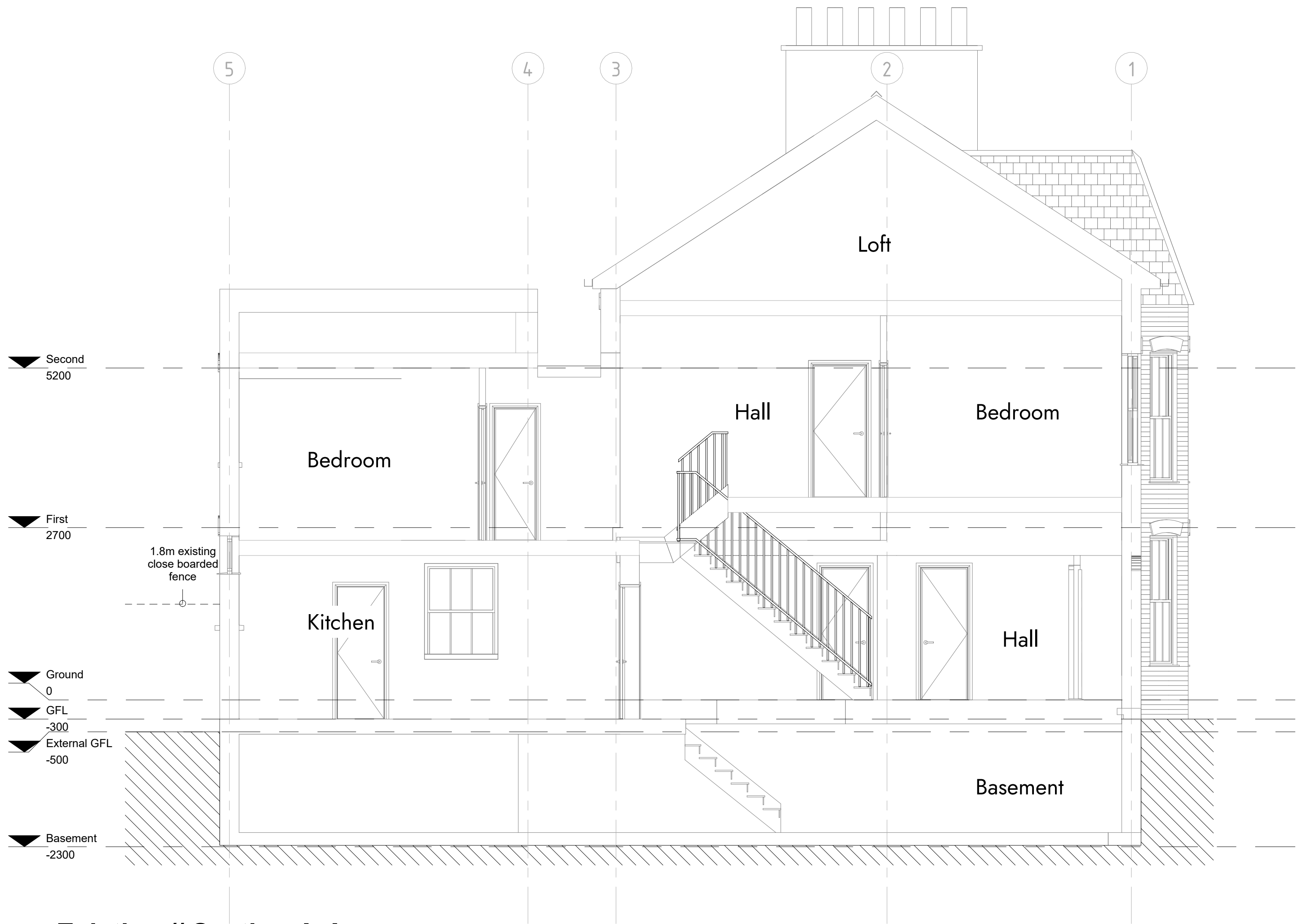
1 Existing // Section A-A 1 : 50
