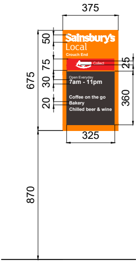
06 WELCOME MESSAGE P 94621 213 1:25@A3
