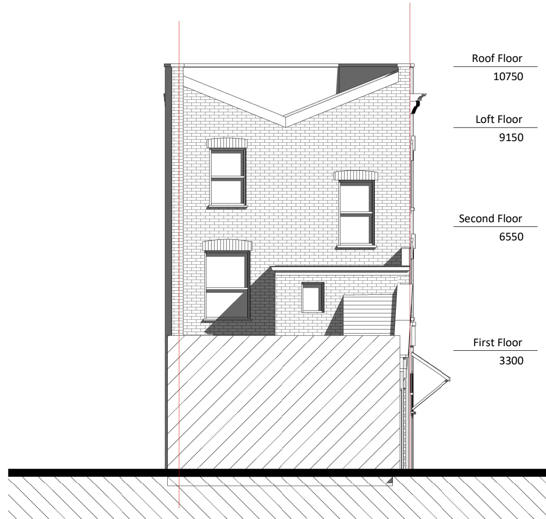
2 Rear 1 : 100
