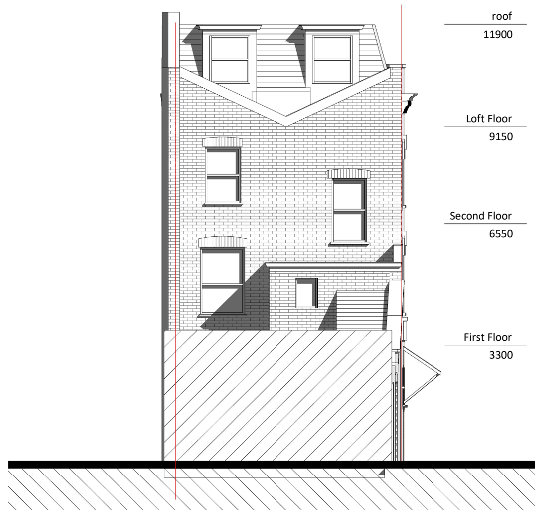
2 Rear 1 : 100
