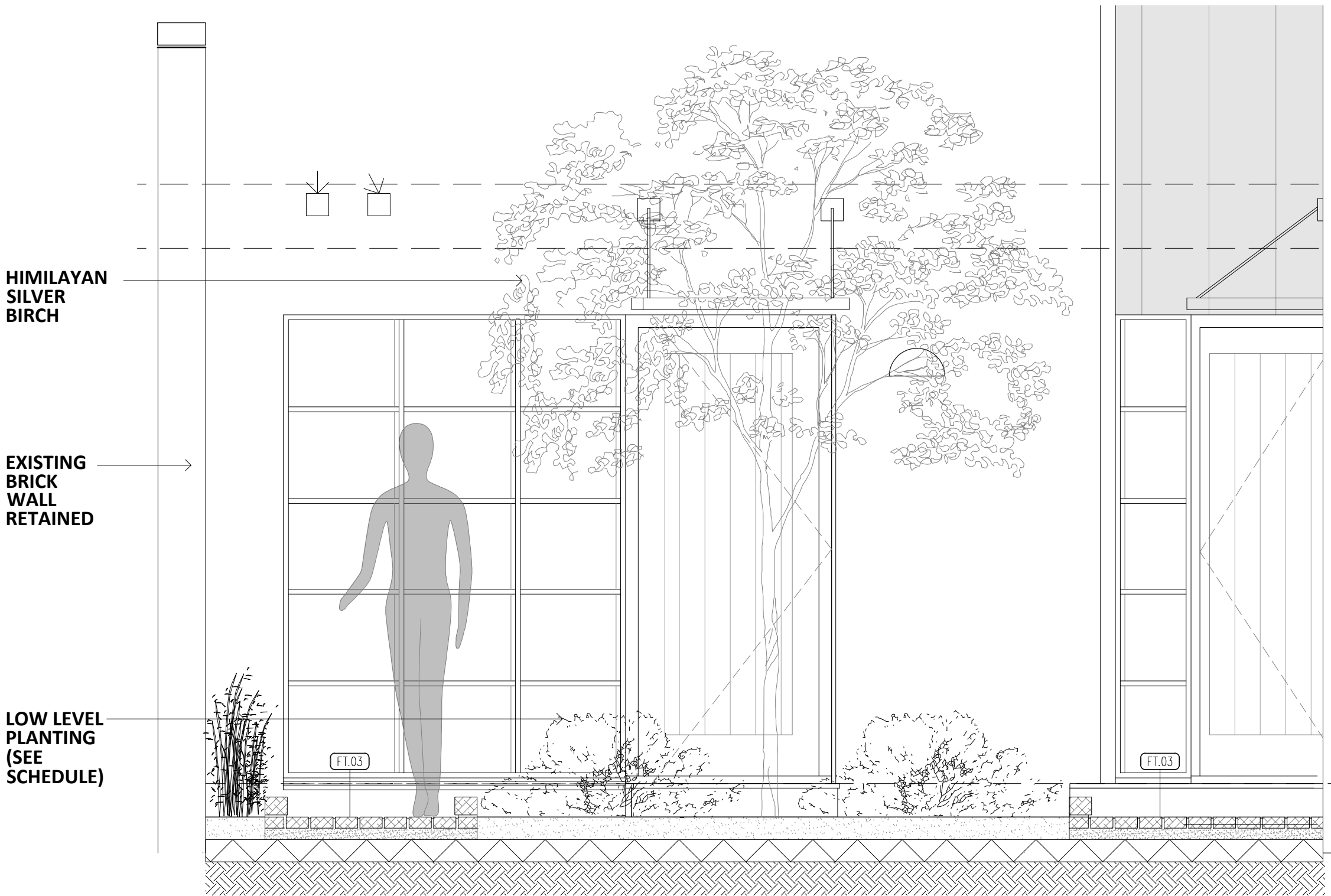
SECTION A-A
