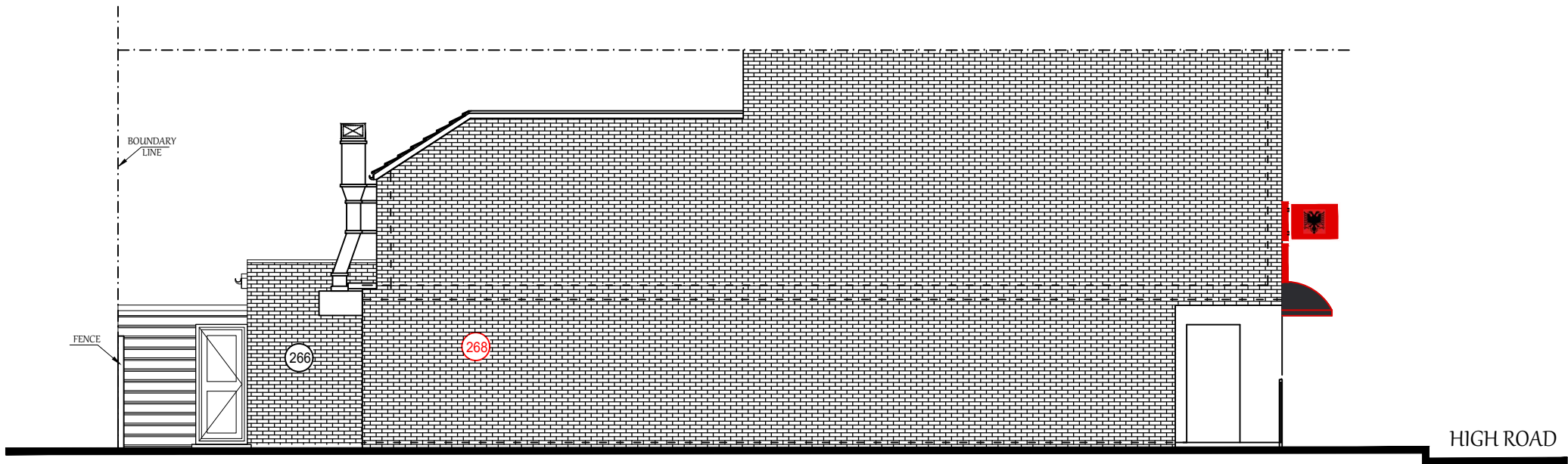
EXISTING SIDE ELEVATION SCALE: 1/100 @A3
