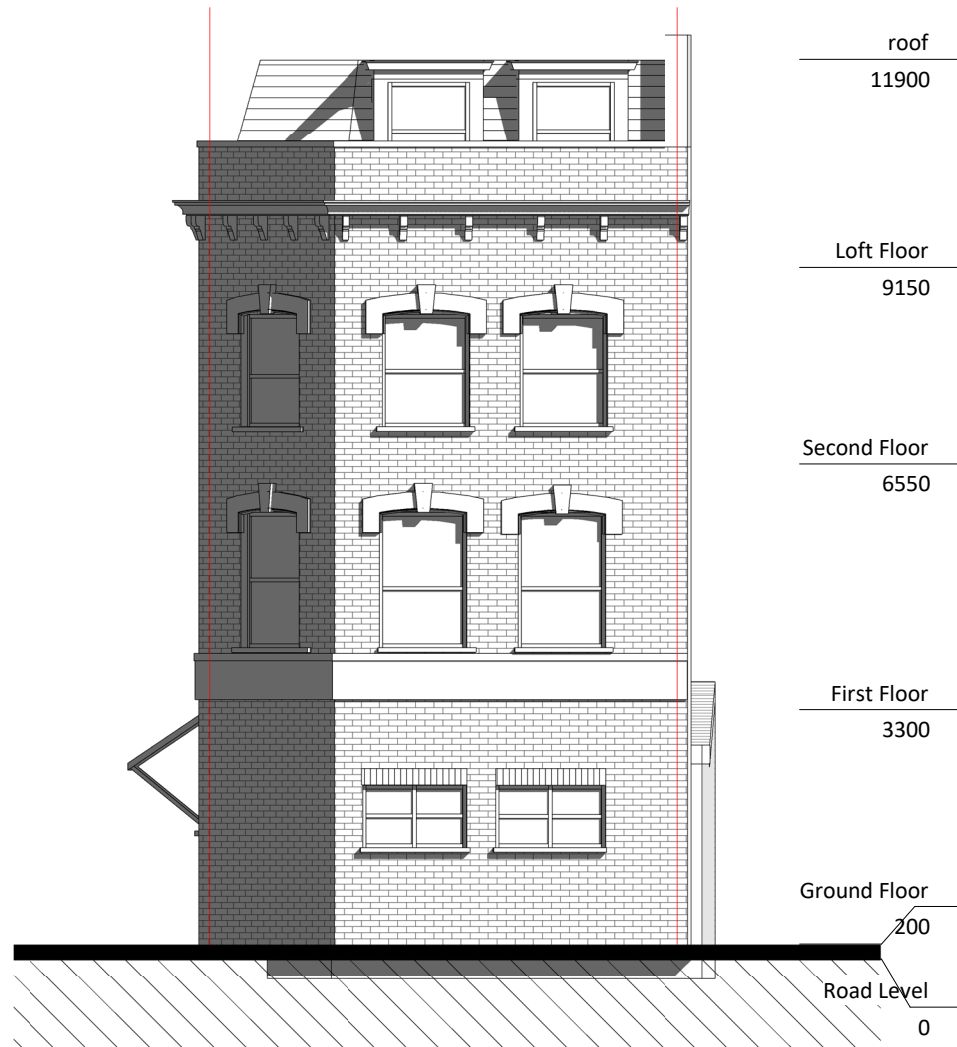
1 Front 1 : 100
