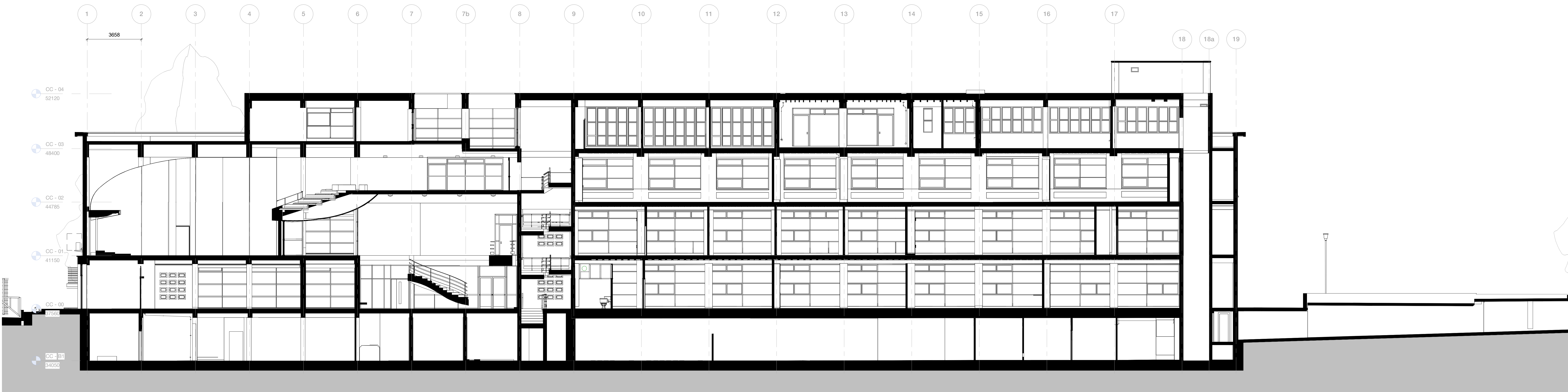
Existing Section BB 1 : 100
