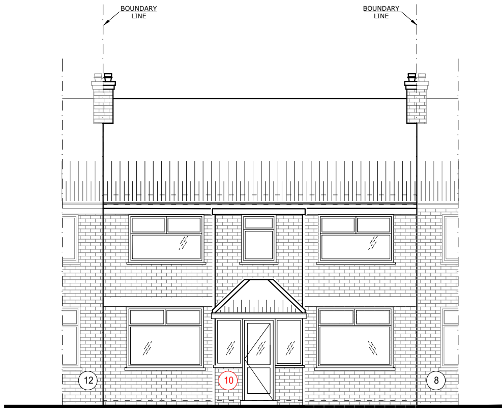
EXISTING FRONT ELEVATION SCALE: 1/100 @A3
