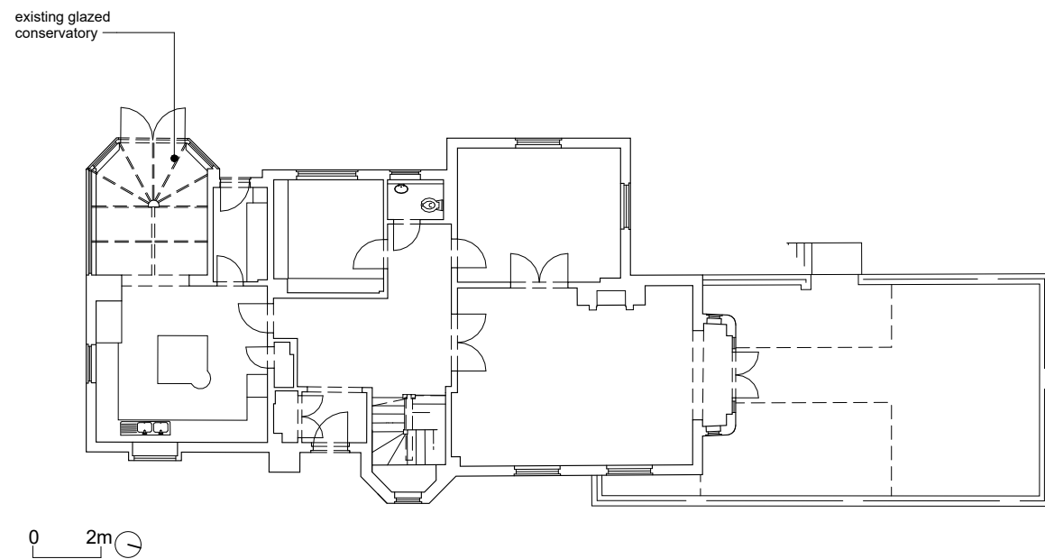
3 Level 0 existing 1 : 200
