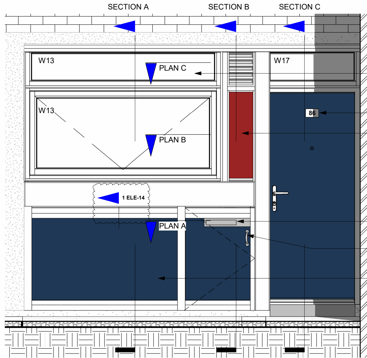
W13 & W17 ELEVATION
