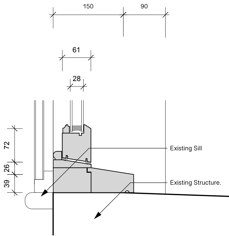
D8 Sash Window - Jamb Detail Scale: 1:5
