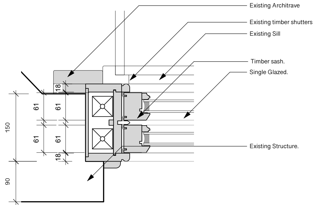
D6 Sash Window - Jamb Detail Scale: 1:5
