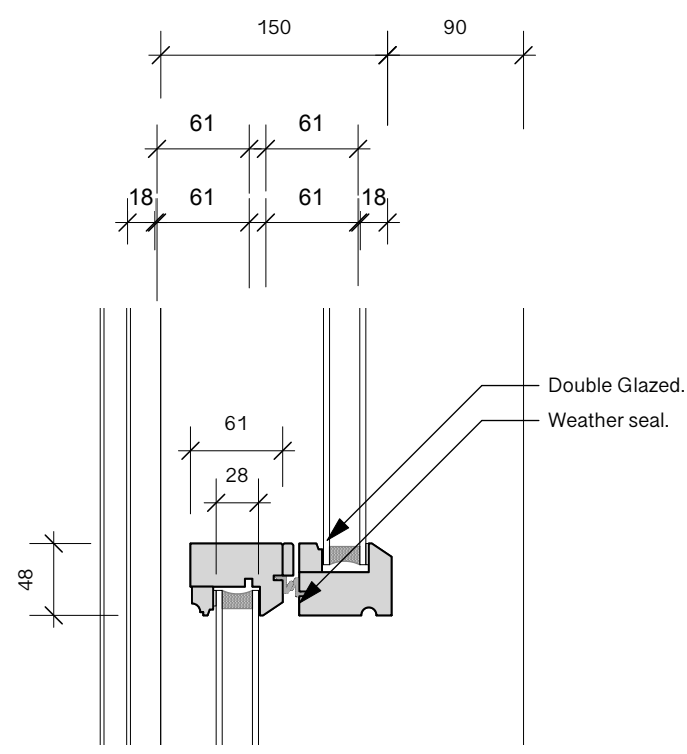
D7 Sash Window - Jamb Detail Scale: 1:5
