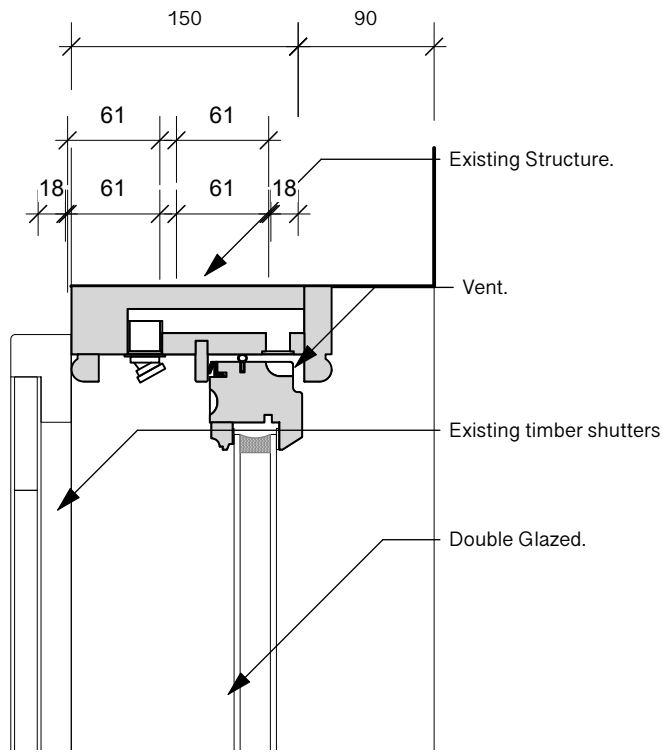
D6 Sash Window - Jamb Detail Scale: 1:5
