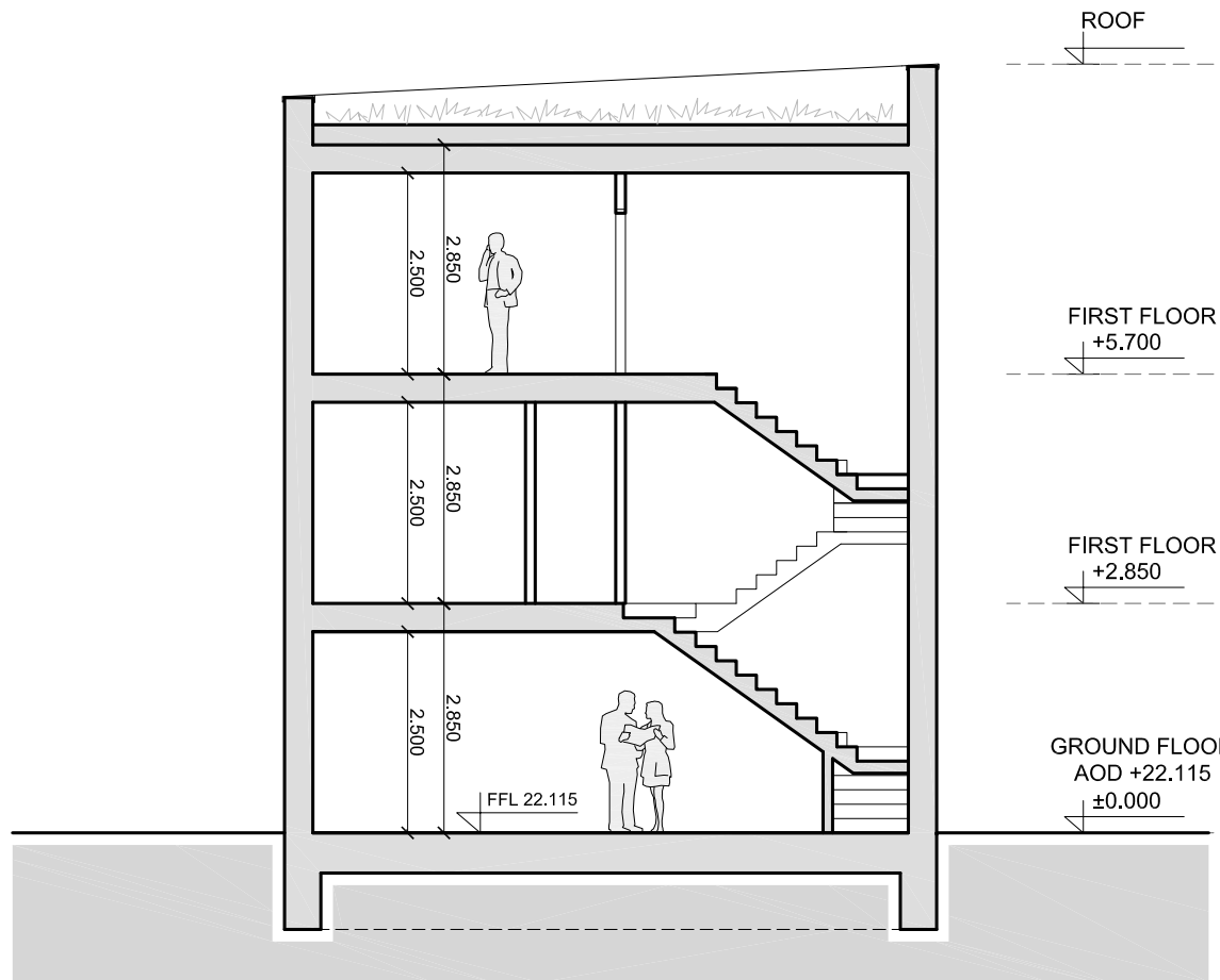
Section A-A
