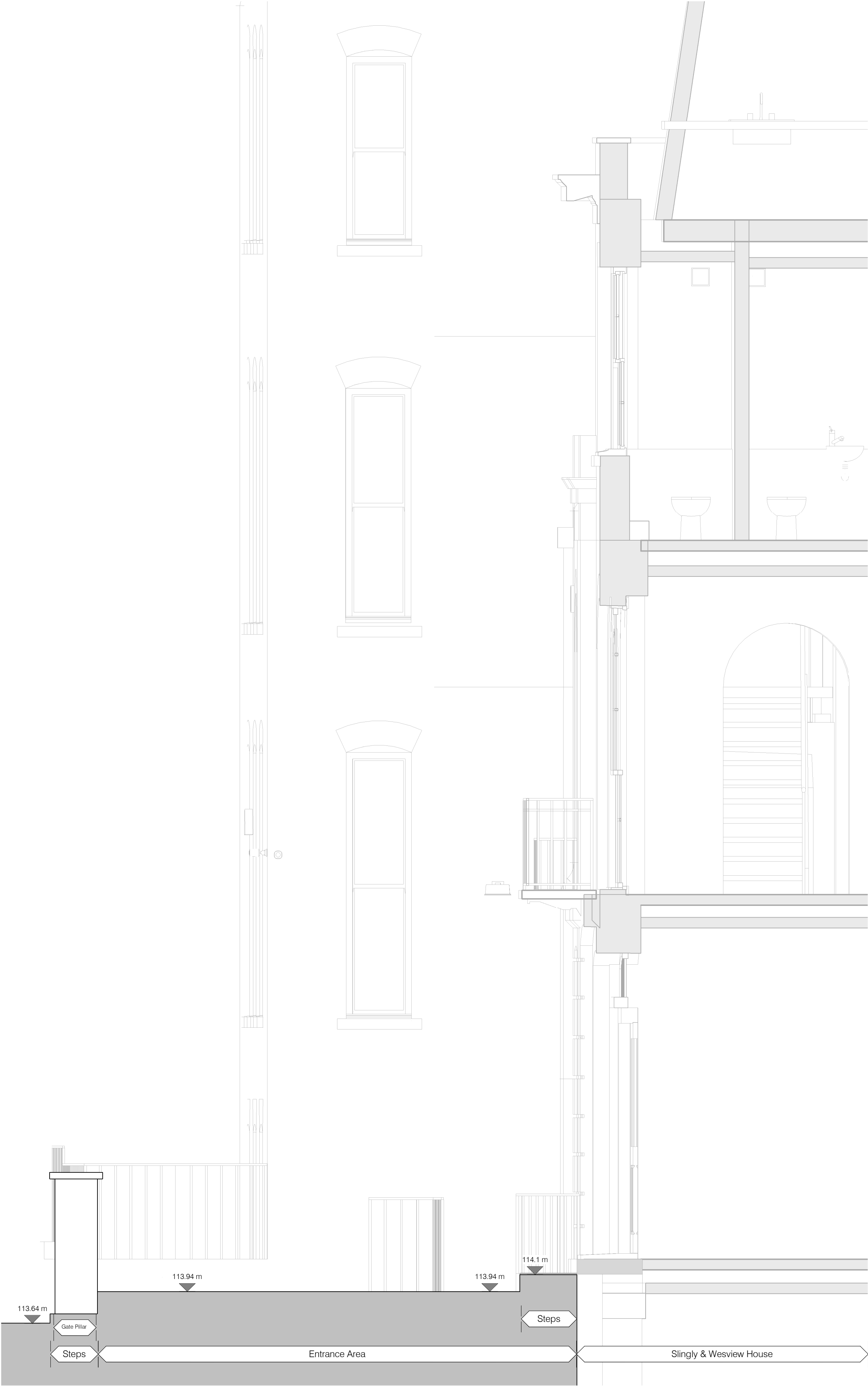
Existing Site Section A-A. 1:25
