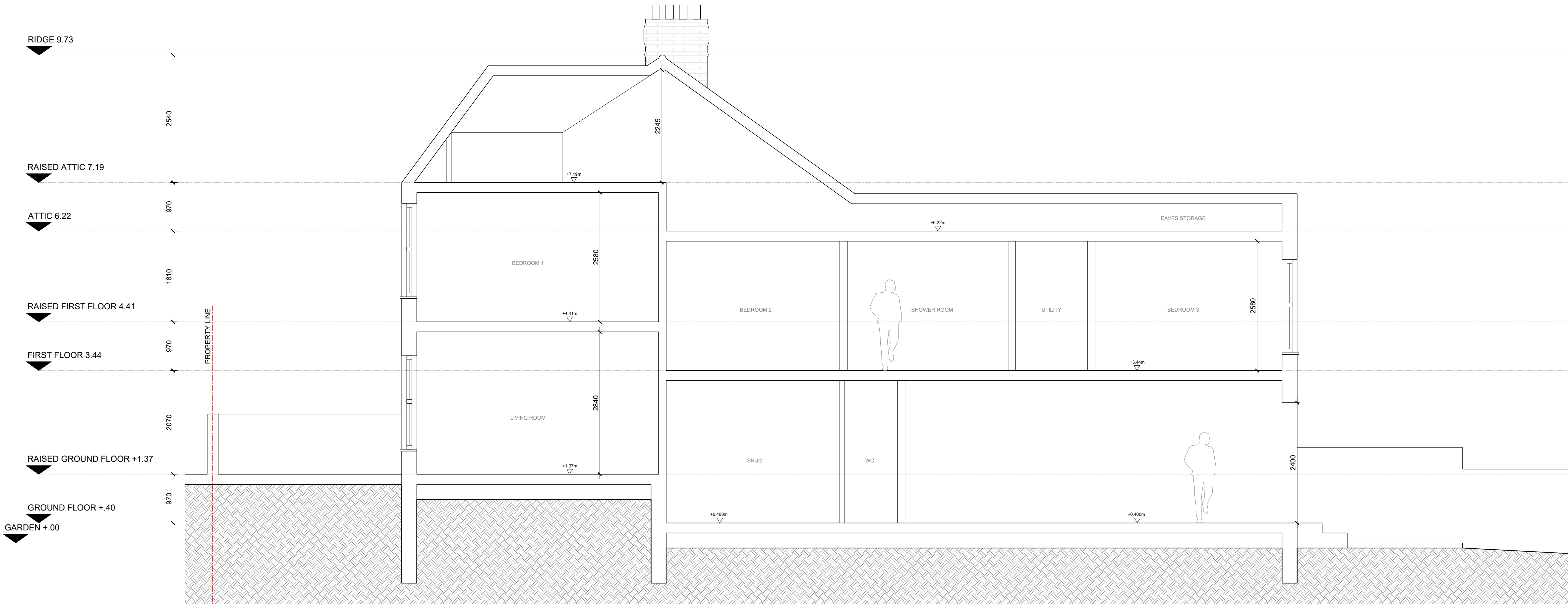
1 EXISTING SECTION 1 : 50
