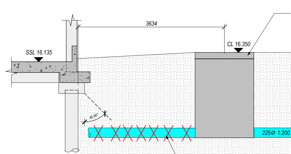
SECTION 1:50 S3 CV-2115
