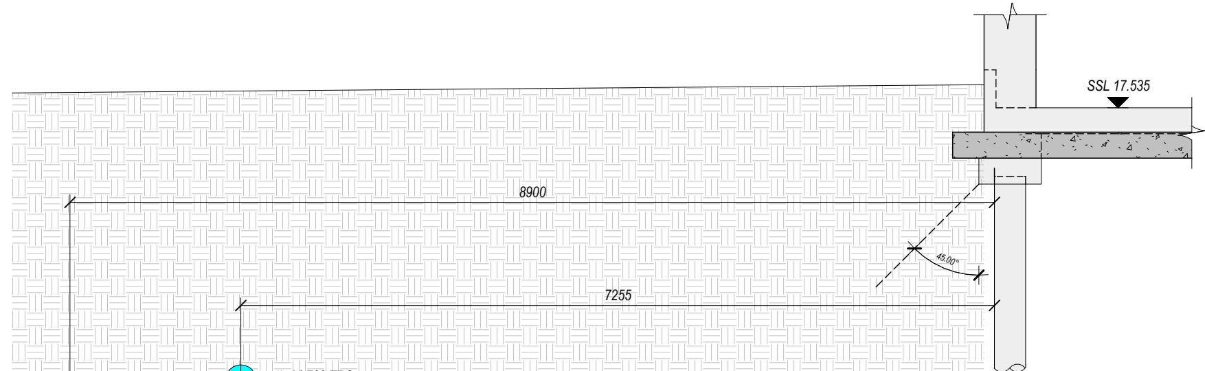
SECTION S4 1:50 CV-2111
