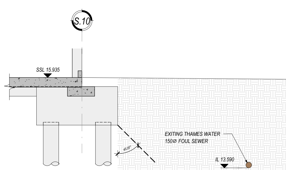
SECTION S2 1:50 CV-2116
