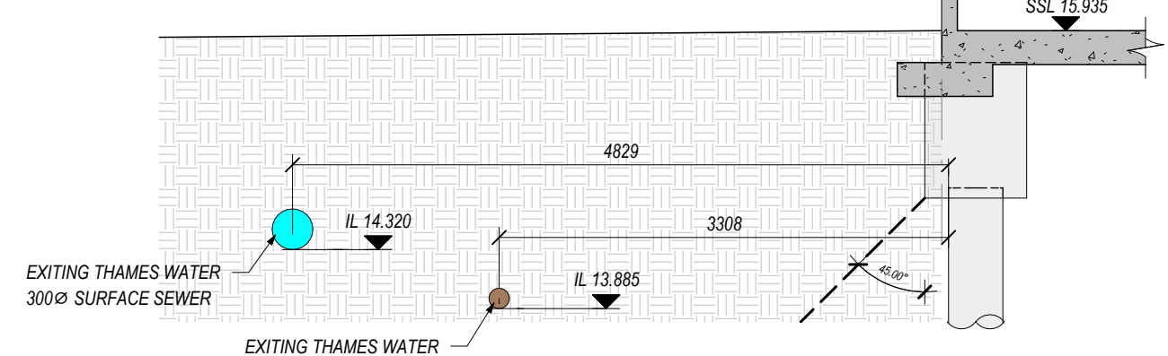
SECTION 1:50 S1 CV-2113
