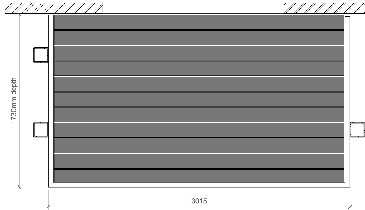
2 Balcony Type 2 1 : 20
