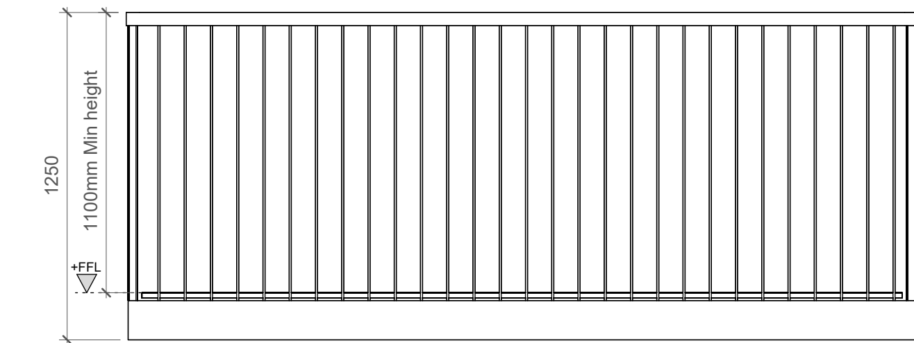
6 Balcony Type 2 1 : 20
