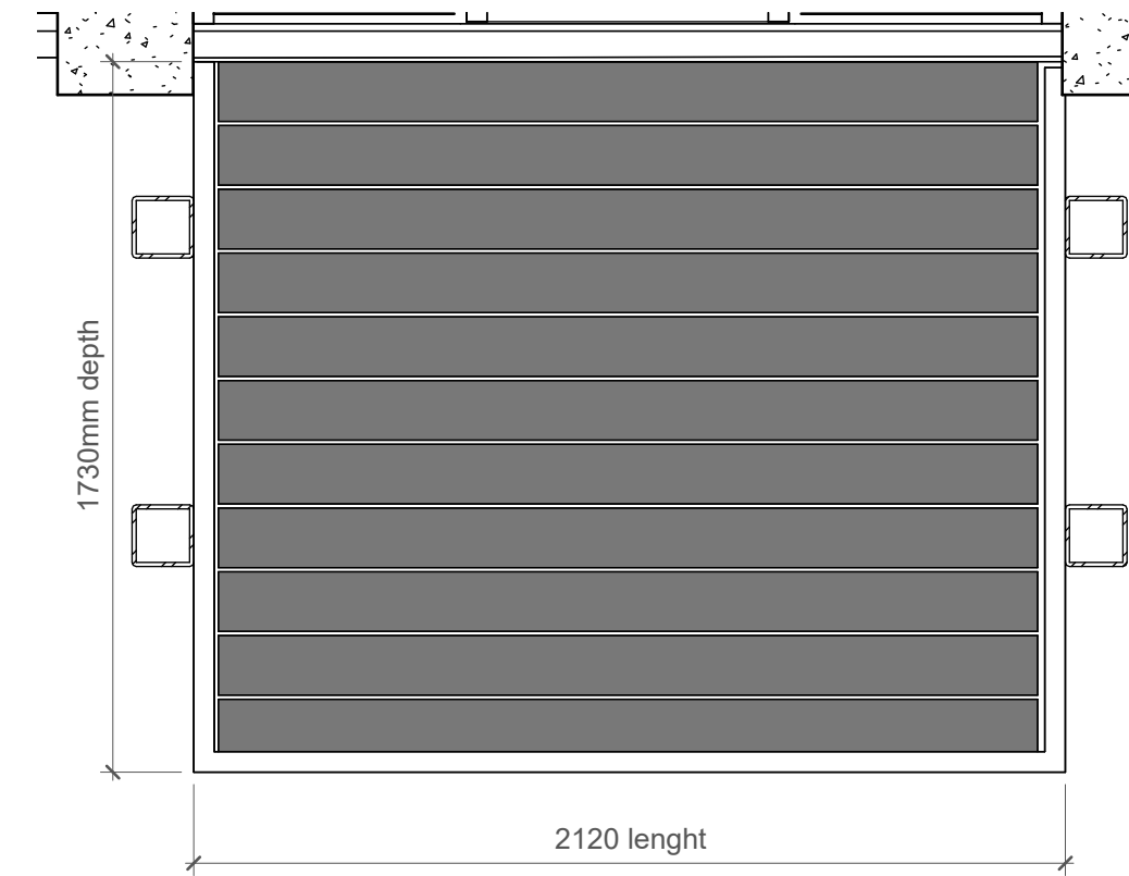
4 Balcony Type 4 1 : 20
