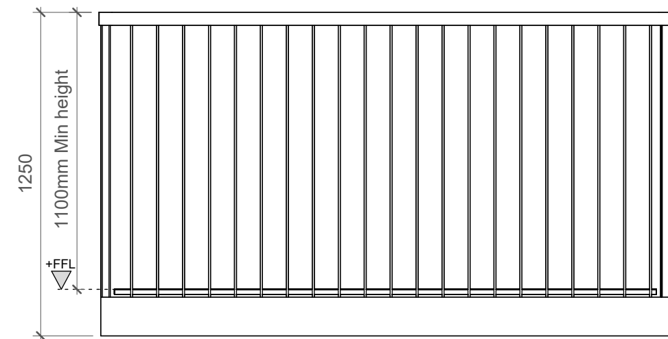
7 Balcony Type 3 1 : 20
