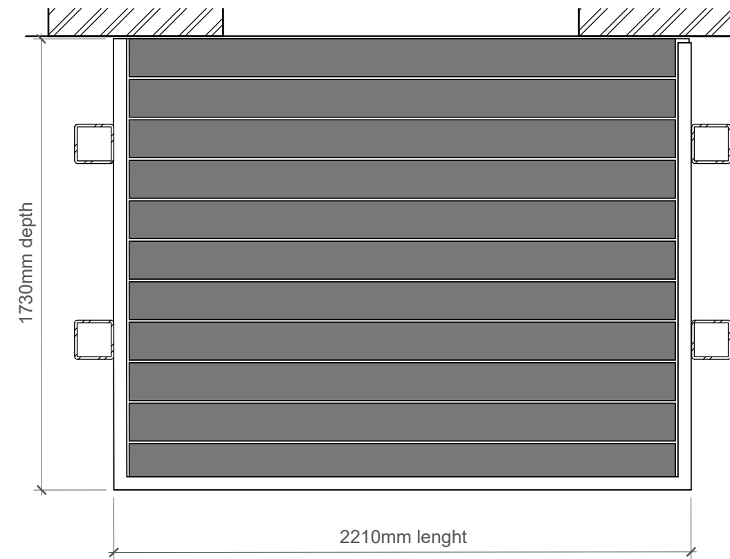
3 Balcony Type 3 1 : 20
