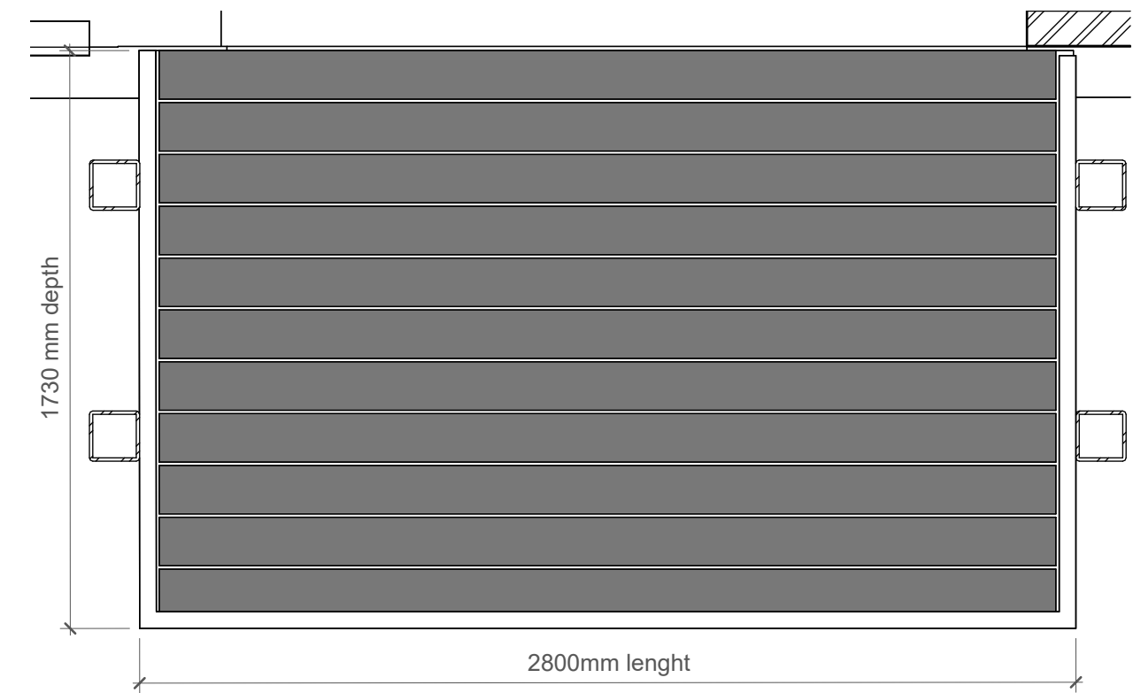
1 Balcony Type 1 1 : 20
