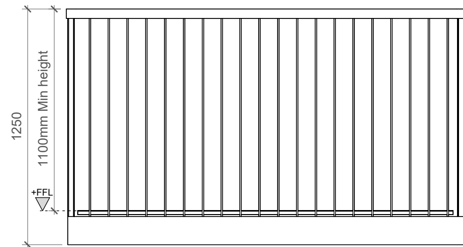
8 Balcony Type 4 1 : 20
