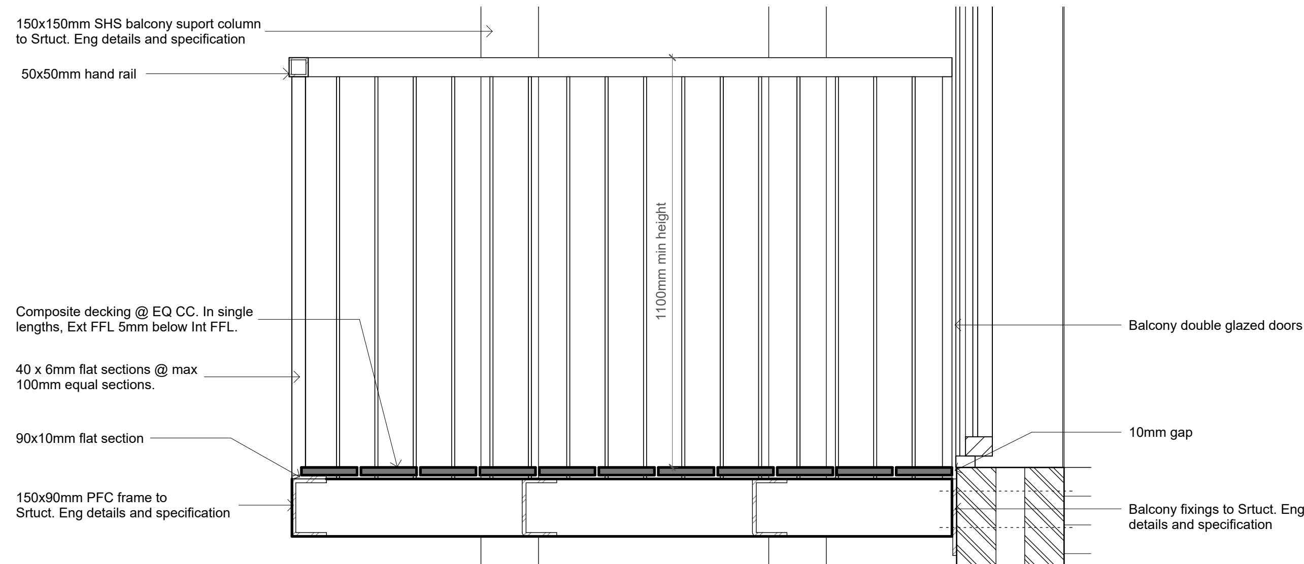
9 Balcony Section AA 1 : 10
