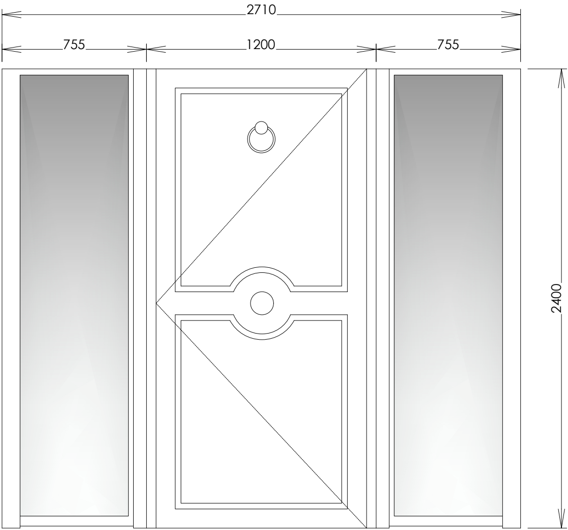
DOOR ELEVATION 1:20
