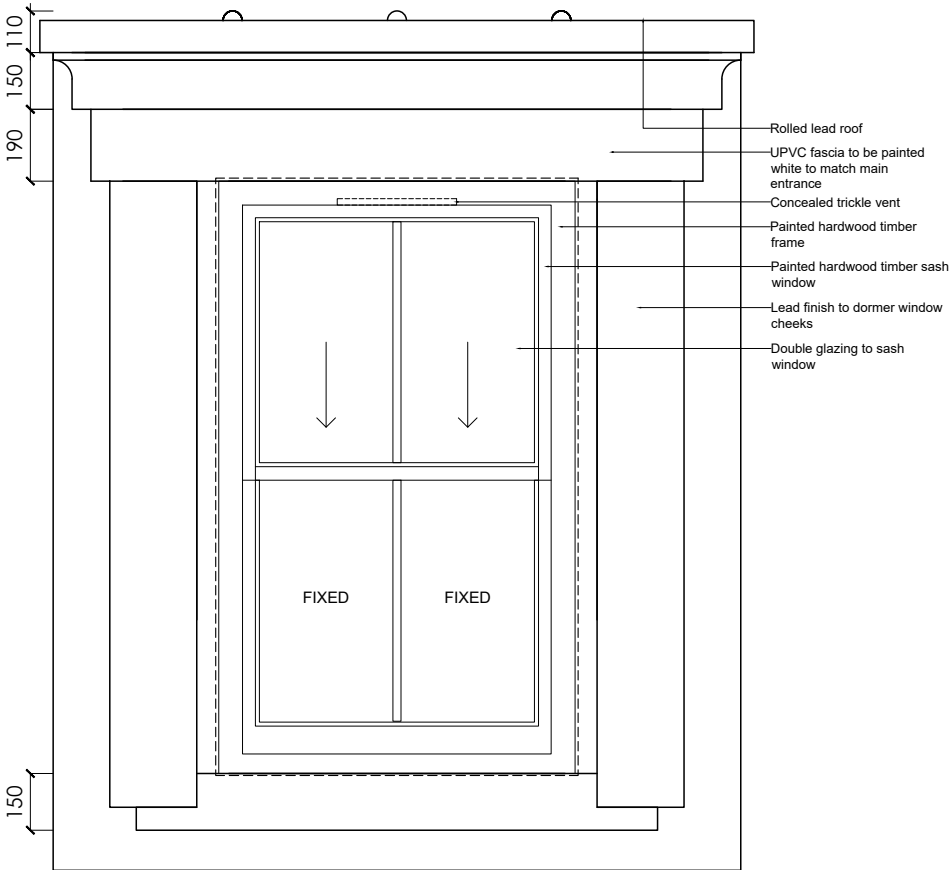
Elevation View Scale: 1:20
