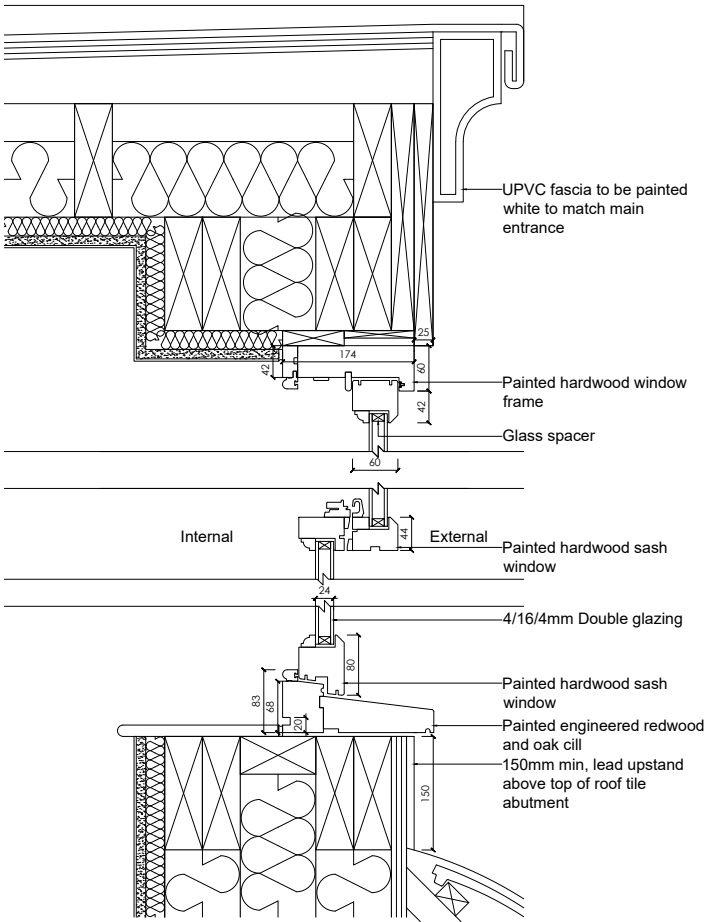
Section Detail Scale: 1:10
