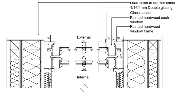
Plan Detail Scale: 1:10
