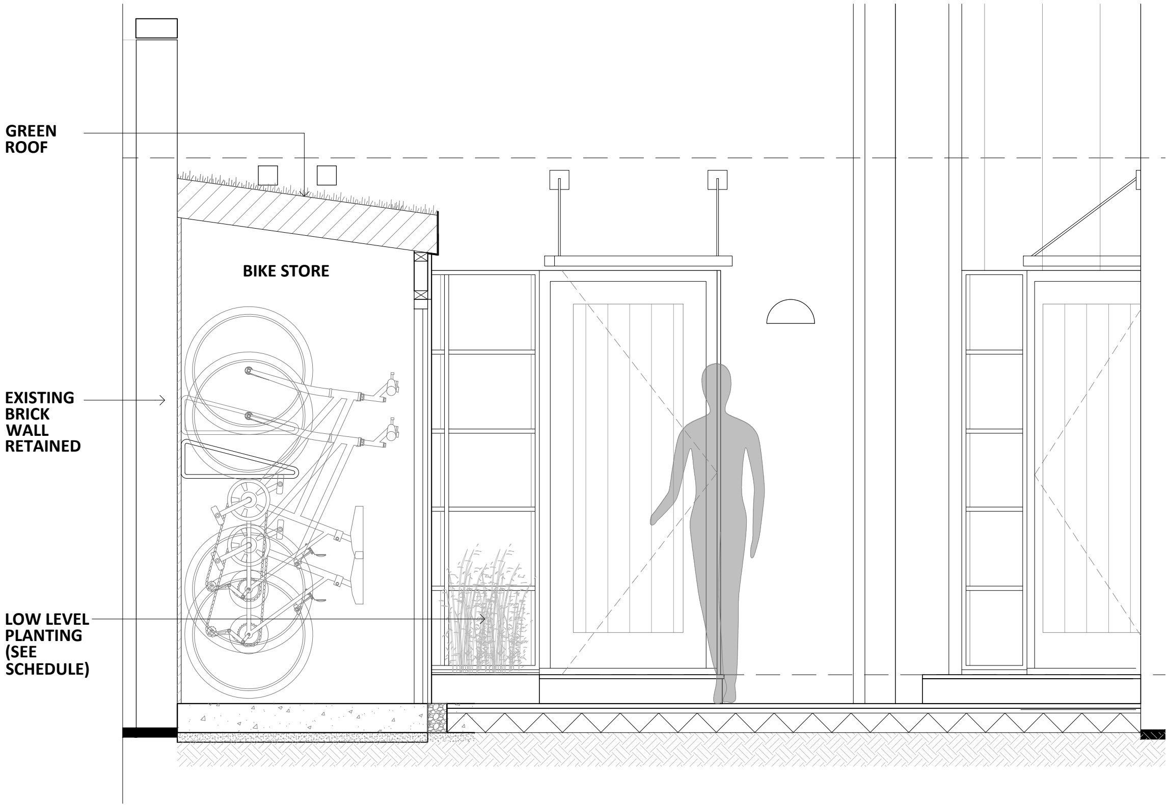
SECTION A-A
