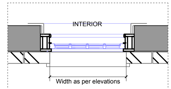
D 1:20 Section A-A
