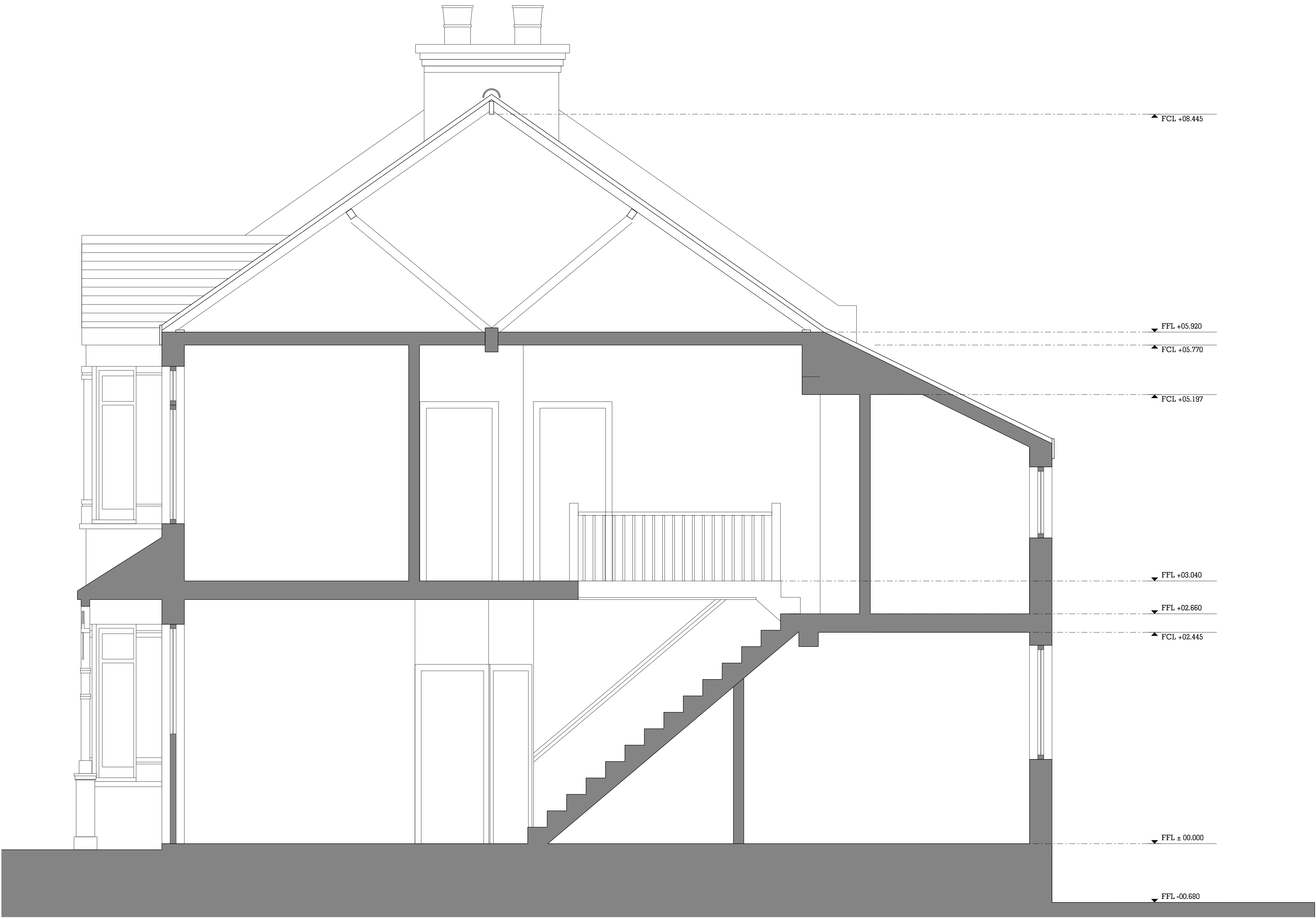
01 Existing Section AA 1:50 @ A3
