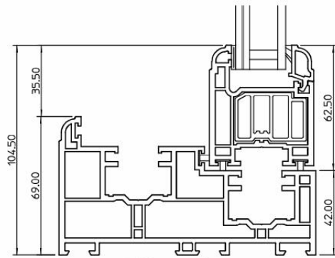
Side Jamb
