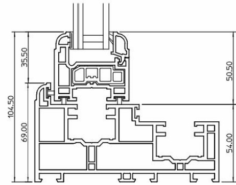
Top Jamb
