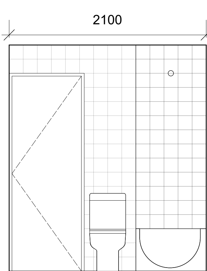
ELEVATION A
