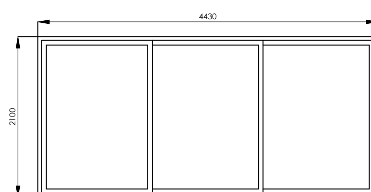
DOOR DETAILS
